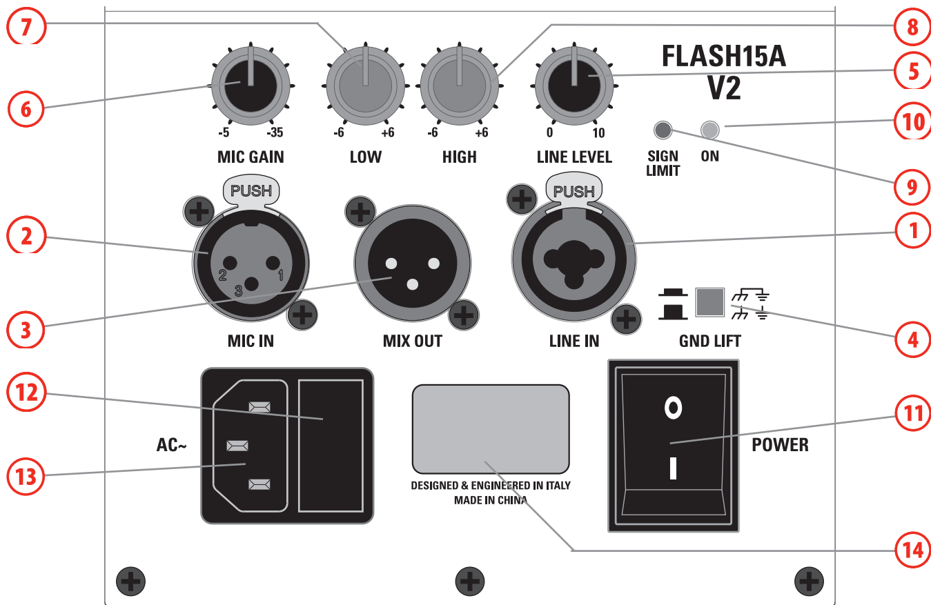
FLASH15A لوحة التحكم (الشكل 1)
